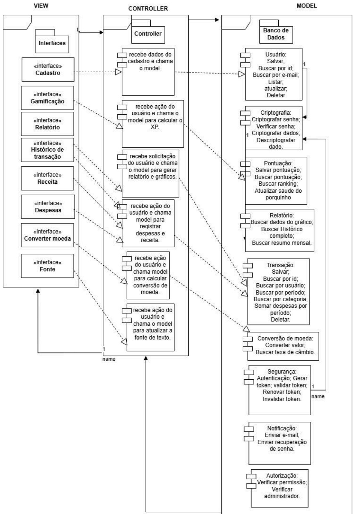
Imagem: Diagrama de pacotes.Fonte: Autoria Própria.
